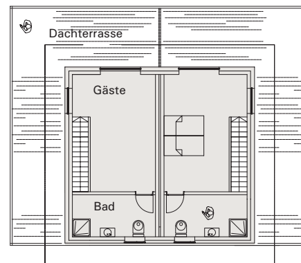
STAFFELGESCHOSS
